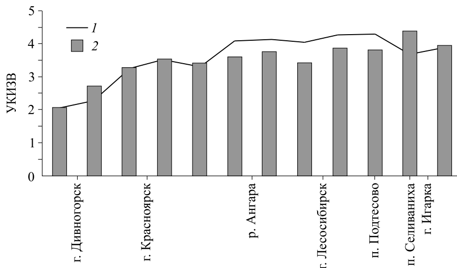
Рис. 3. Величина УКИЗВ в Енисее на участке от плотины Красноярской ГЭС до Игарки в 2010 г. (1) и 2011 г. (2).
